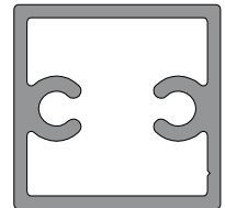
Barrote CUADRADO 30 mm.
