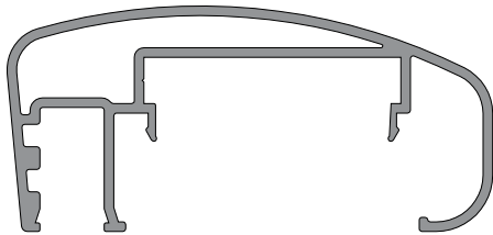
Pasamanos ELÍPTICO CRISTAL
